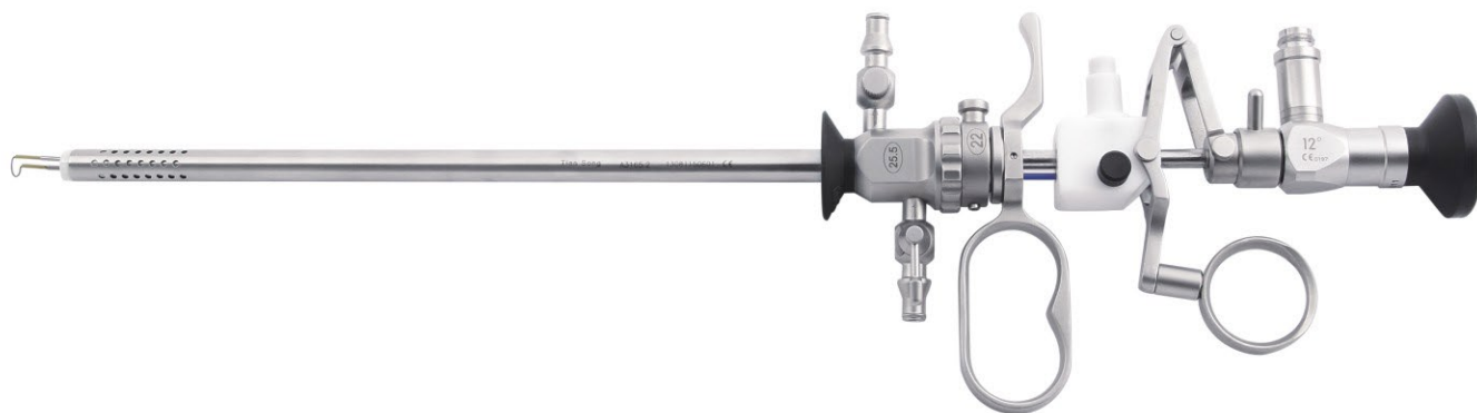
A0011 12° 内窥镜 Endoscope Φ4×302mm
