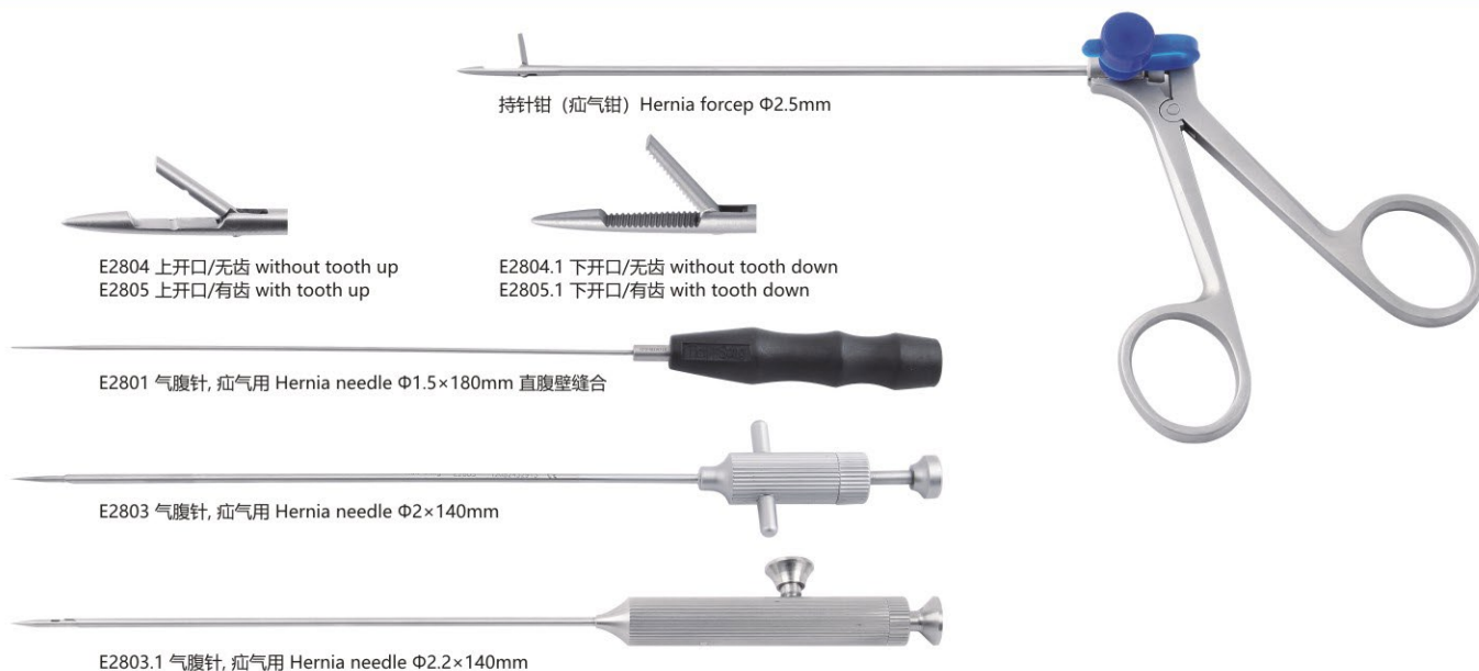
E2803.1 气腹针，疝气用 Hernia needle Φ2.2×140mm
